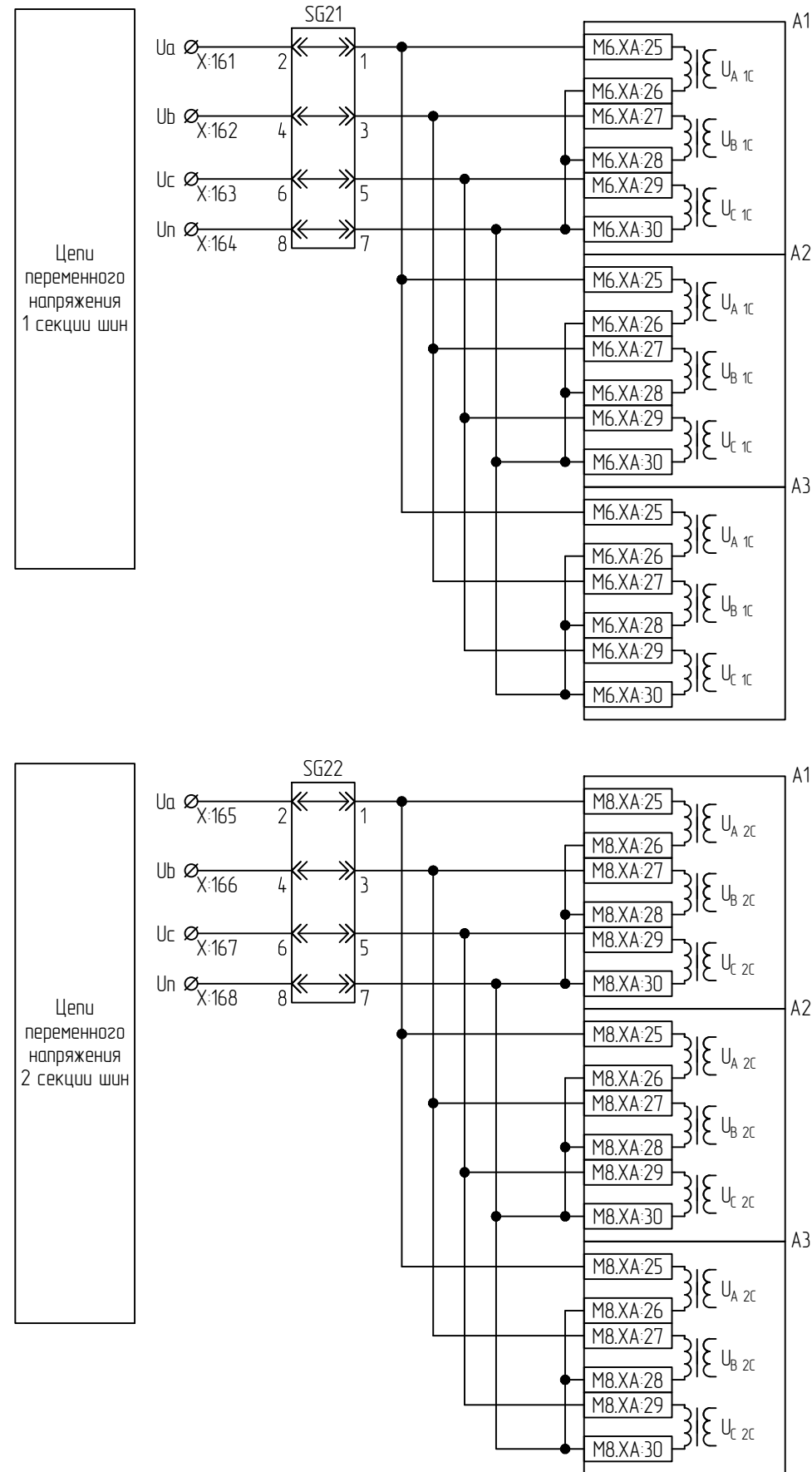
Цепи переменного напряжения
