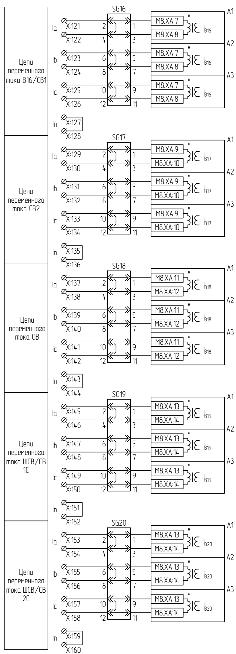
Цепи переменного тока
